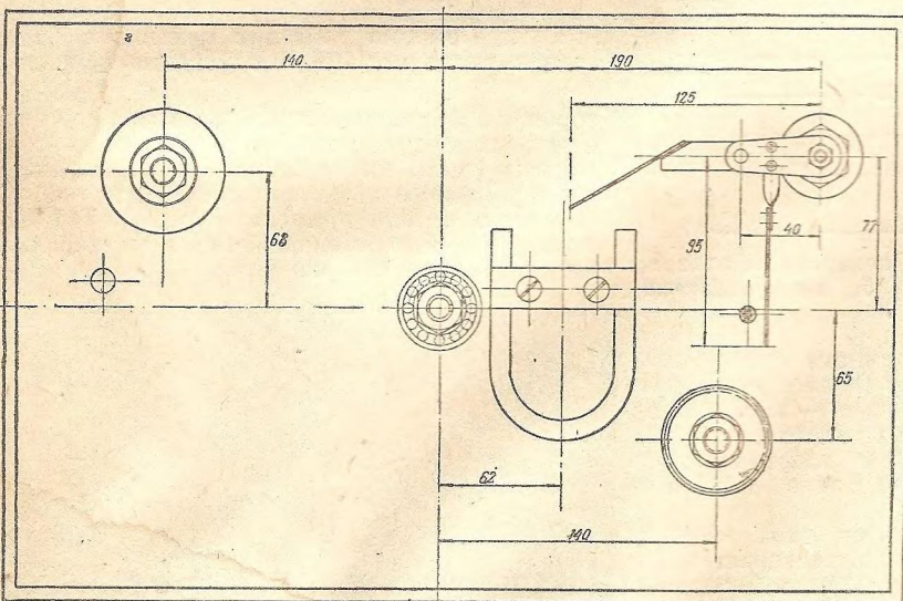
Рис. 15. Верхняя доска автомата (вид снизу). Видны места установки стенок, упорный шарикоподшипник диска граммофона, магнит контакта пуска мотора и поводок поворота тонарма с контактами и установками на пластинки типа «Гигант». Около пружинки установки тонарма виден винт, задерживающий ее при работе с пластинками типа «Гигант»
