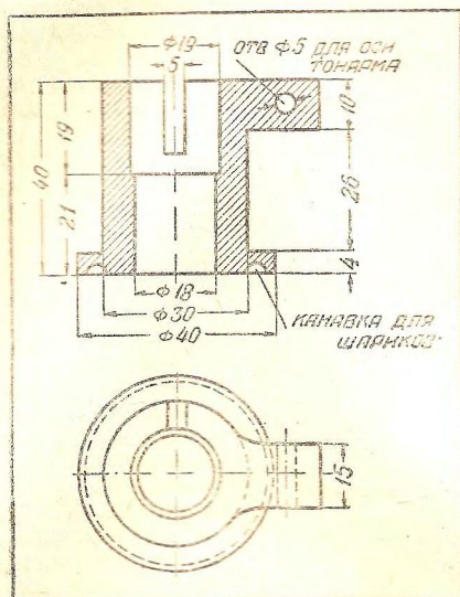
Рис. 10. Поворотная головка стойки тонарма. В отверстие для оси тонарма помещается его горизонтальная ось, а в вертикальном отверстии (рис. 9) проходит шток подема адаптера. В продольном прорезе находится шпилька штока, предохраняющая его от проворачивания в головке стойки при повороте адаптера
