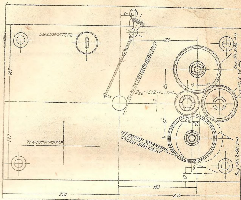
Рис. 16. Нижняя доска автомата (вид снизу). Расположение шестерен механизма автомата и установка его для работы с пластинками типа «Гранд» и «Гигант»
